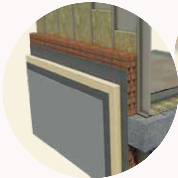
Sistema SATE
