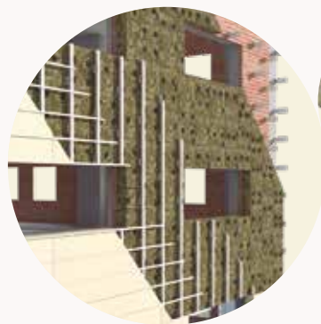
Fachada ventilada
