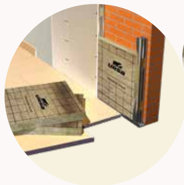
Trasdosado en fachadas y medianeras
